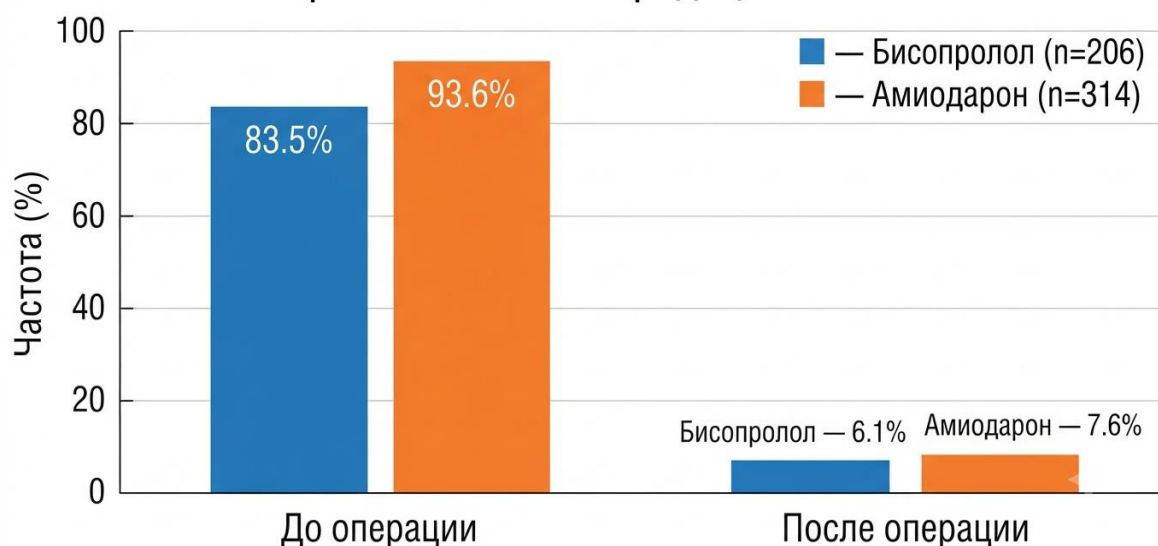
Рисунок 1. Динамика частоты желудочковой экстрасистолии III–V градаций по Lowen до и после операции в подгруппах бисопролола и амиодарона.
